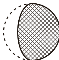
gibbous moon
